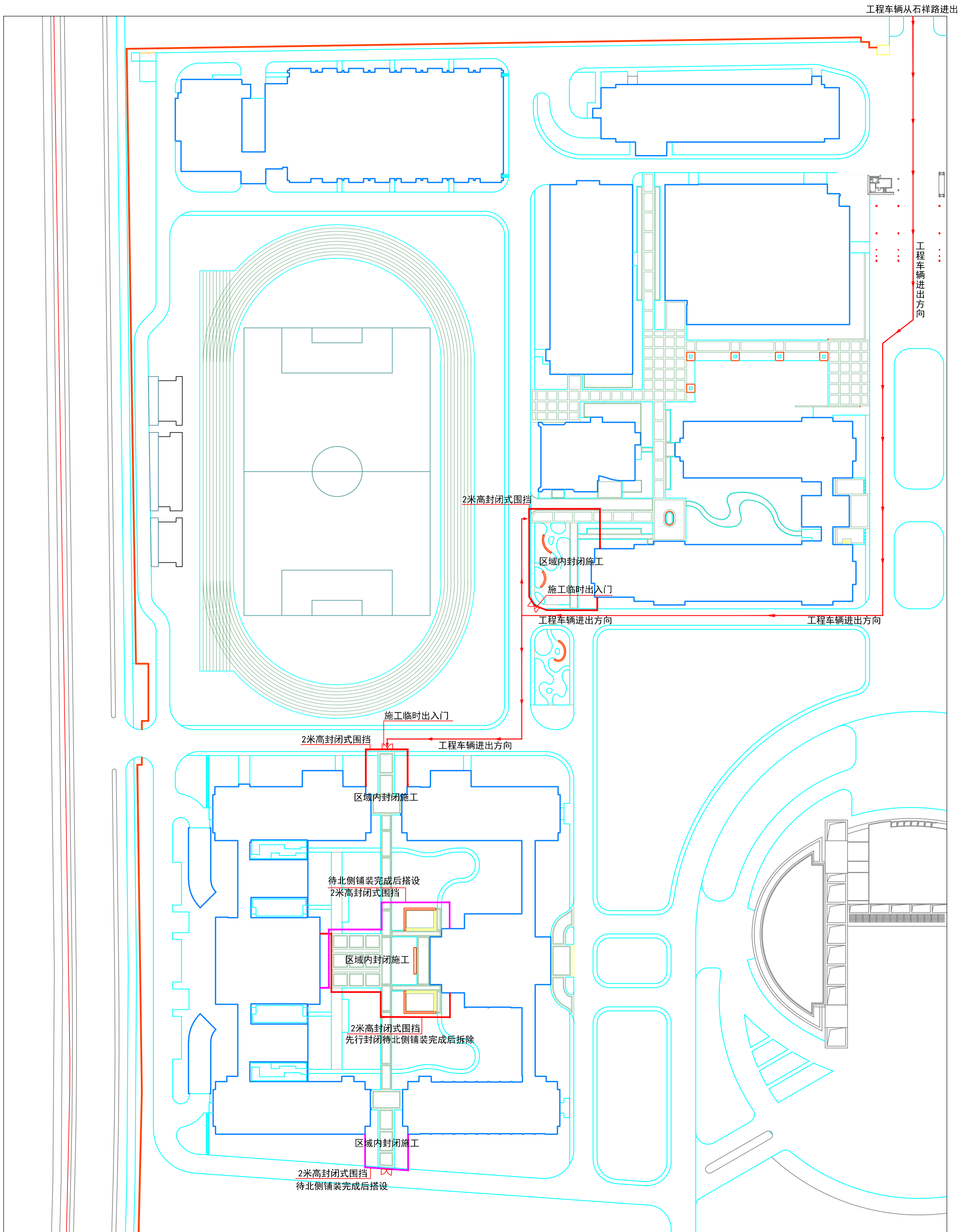
施工临时围挡及车辆通行布置图
